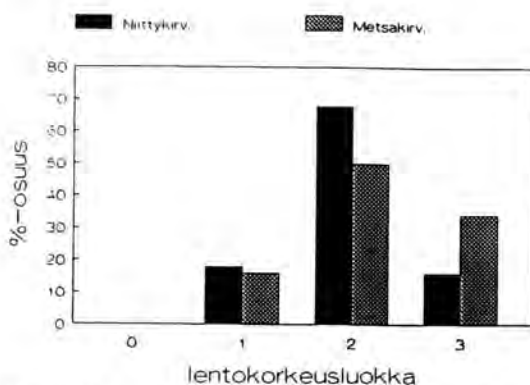
Kuva 6. Muuttotarvien lentokorkeusjakaumat. Lentokorkeusluokat: 0 = puusta puuhun, 1 = 0...10 metriä, 2 = 10...50 m ja 3 yli 50 m.
